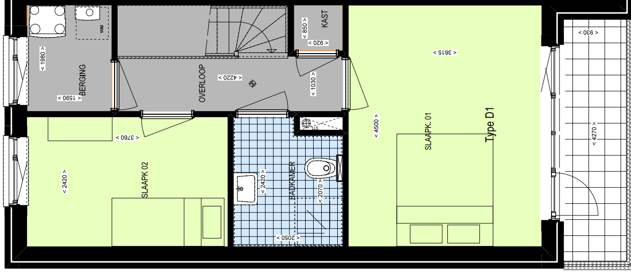
2e Verdieping
